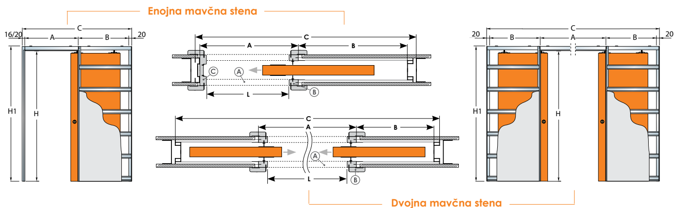
HEMA PODBOJA VRAT ZA DRSNI SISTEM (sistem mavčnih sten)
